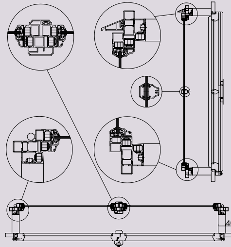
Schnitt Außenöffnend
