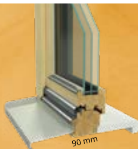
LIGNUM I Holzfenster Bautiefe 90 mm (3-fach verglast)
