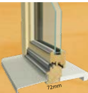
LIGNUM I Holzfenster Bautiefe 72 mm (2-fach verglast)
