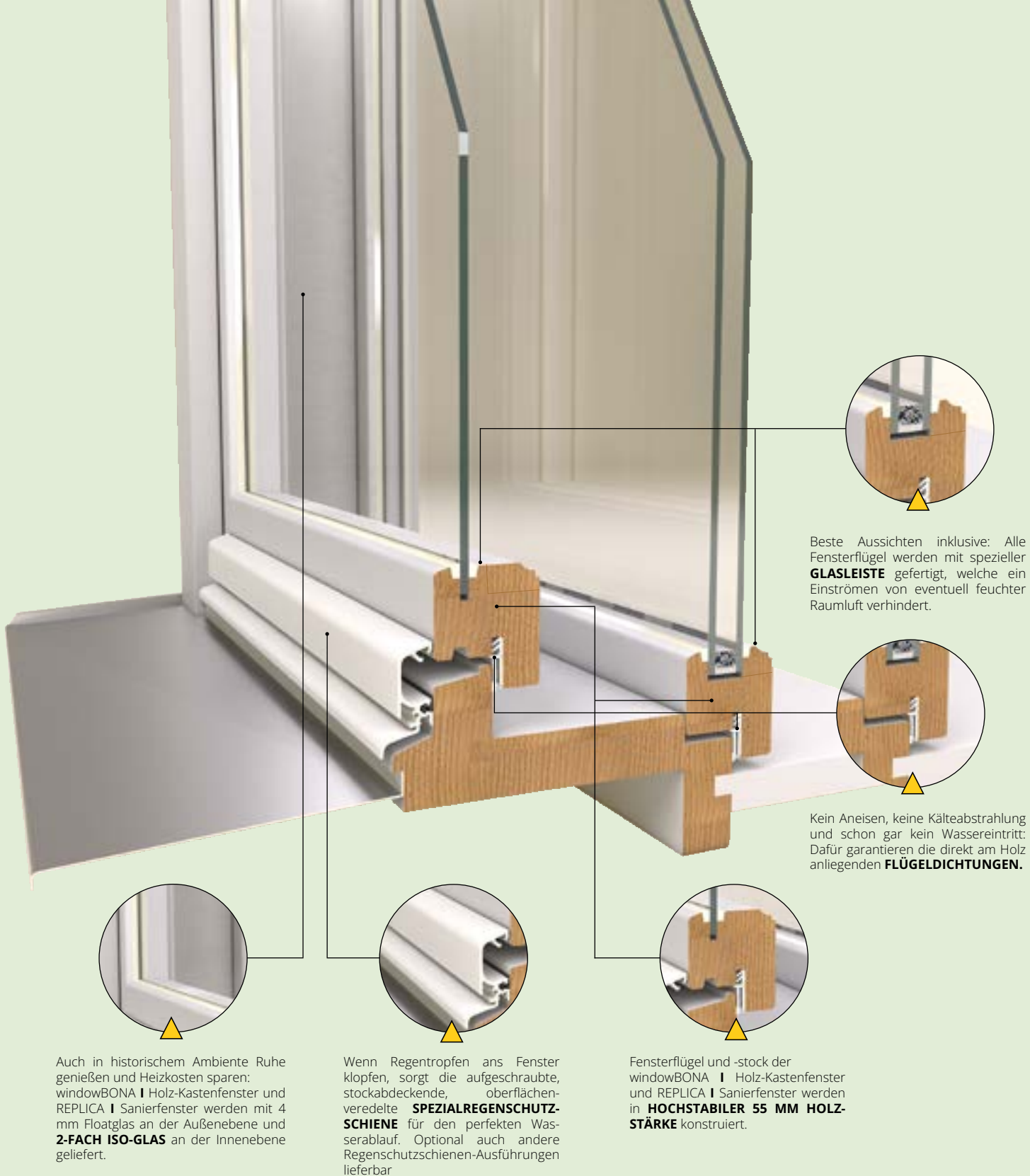
REPLICA I Sanierfenster Abbildung: Außenebene
